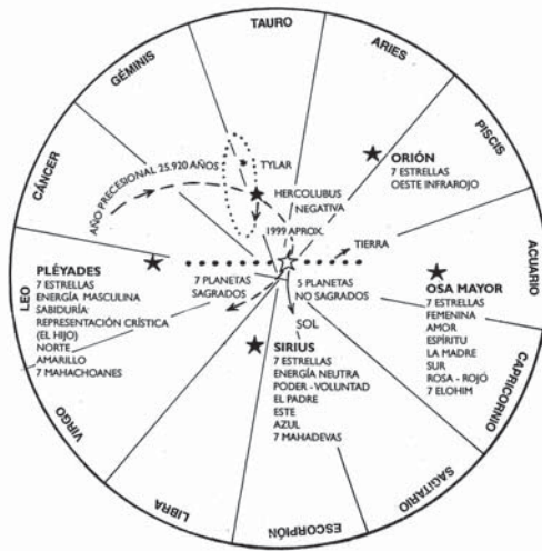
Fig. 7.- La Rueda Giratoria en términos astrológicos y esotéricos es el esquema que indica el fenómeno de la Precesión. Según la astrología, para 1999 aproximadamente estaremos en la Era de Acuario; estos cálculos varían según los investigadores.
