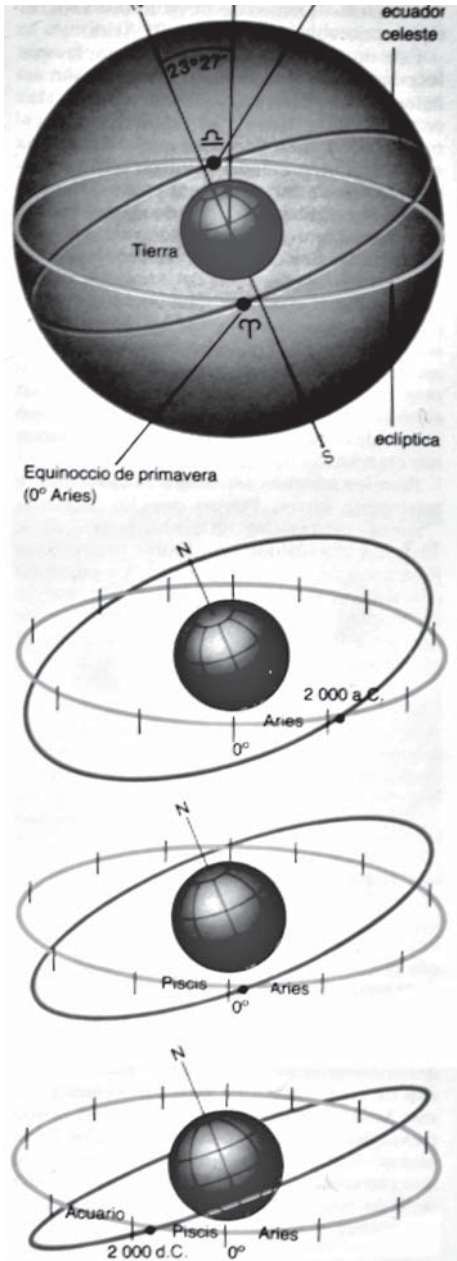
Fig. 10.- Los equinoccios de Primavera y Otoño son aquellos dos días del año en que el día y la noche tienen igual duración.
