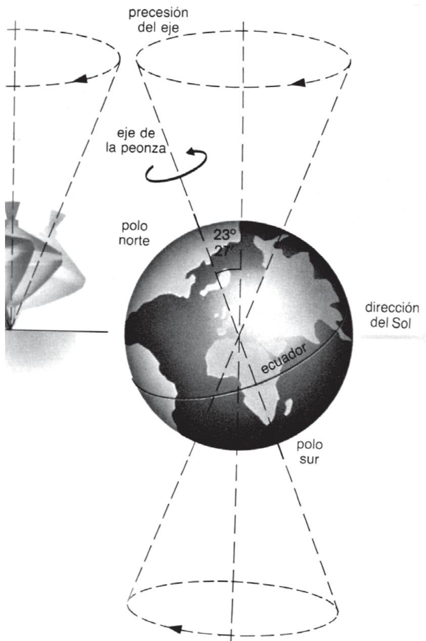
Fig. 9.- La Tierra al girar se "bambolea" como un trompo causando el tercer movimiento, llamado precesión, debido a la fuerza de gravedad del Sol. Los polos y el Ecuador celestes se desplazan con respecto al fondo de estrellas fijas.
