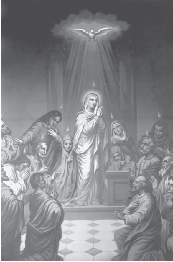
Fig. 77.- La venida del Espíritu Santo sobre los apóstoles y Nuestra Señora el día de pentecostés (cfr. Hechos de los Apóstoles 2, 1-13).
