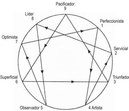
Fig. 122.- El eneagrama es toda una industria de la Nueva Era que se está extendiendo rápidamente, a través de cursos entre católicos, protestantes y de otras religiones. Comunidades religiosas, parroquias, muchos sacerdotes y monjas lo usan para “mejorar su personalidad y orar en sincronía con las vidas pasadas”. Los católicos deben saber que tiene orígenes ocultos, para que su fe en Cristo Jesús no sea contaminada con esta técnica de “cristianismo esotérico”.
